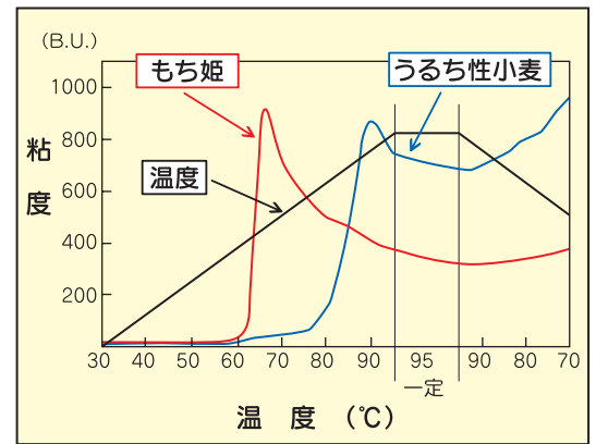
もち小麦の糊化特性(アミログラムの図形)
