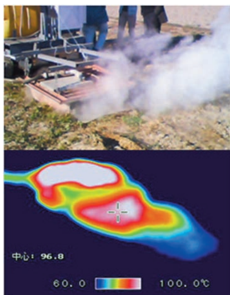
図2 蒸気処理防除機によるほ場表面加熱の様子 サーモグラフィーにより撮影 蒸気噴出部直下の地表温度は90~100℃に達する
