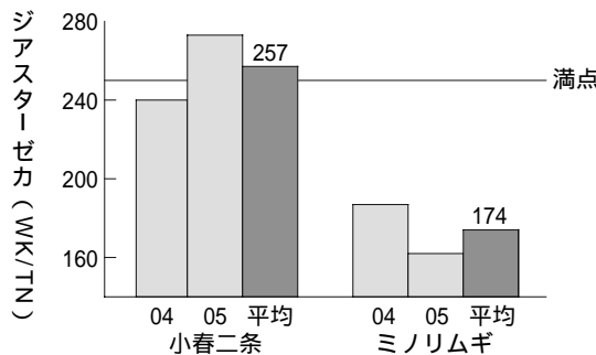
図6 「小春二条」の麦芽蛋白当たりのジアスターゼ力
