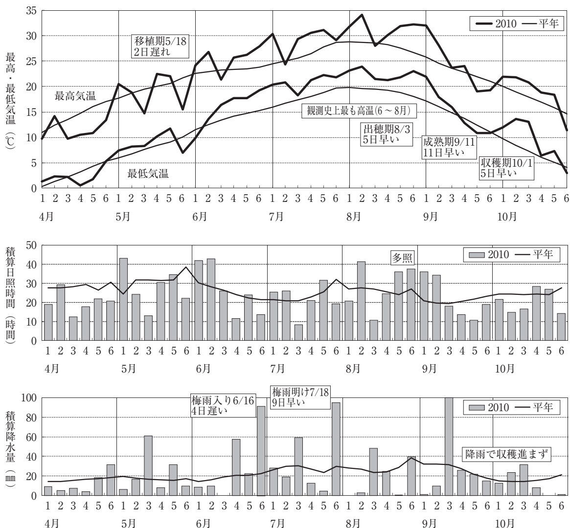
図10 気象経過
