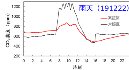
適時CO 2 施用技術による ハウス内CO 2 濃度
