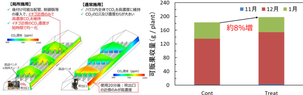
通常施用と局所CO 2 施用下の CO 2 濃度分布(10分後)
