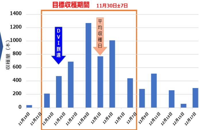
図3 目標収穫日11月30日とする計画出荷実証における日ごとの収穫量(合計6310本、出荷率86%)
