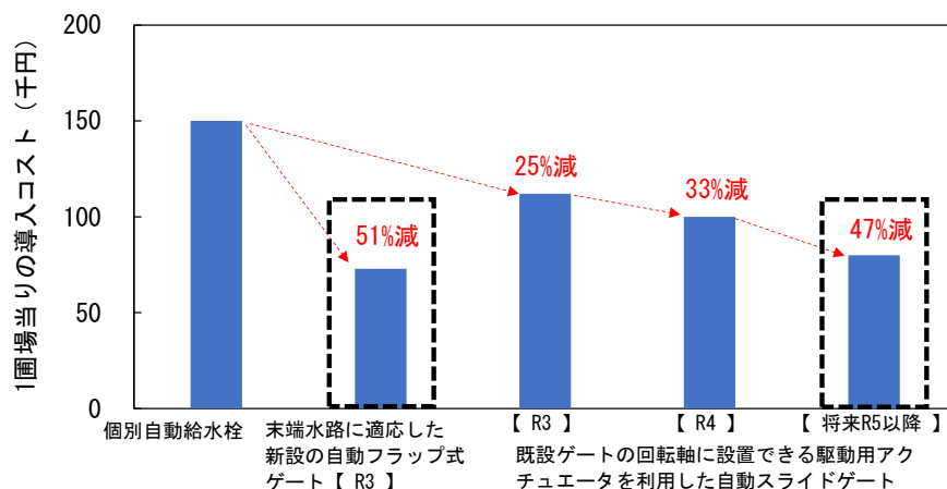
図3 一括給水システム導入によるコスト削減効果
